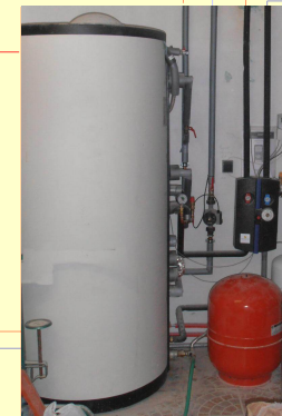
Warmwasser- oder Pufferspeicher Verteilung Steuerung
